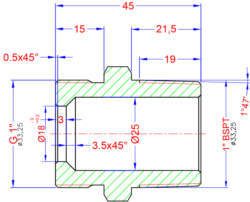
A-A KESİTİ
